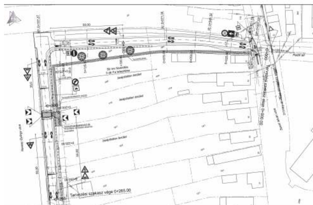
A tervlapon a Hevesy György utca érintett szakaszának tervezett helyszínrajza látható
